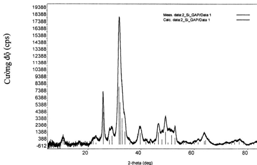
Giản đồ nhiễu xạ XRD của mẫu vật Si-HA với hệ số thay thế silic x=2
