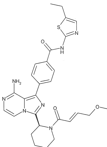
(S,E)-4-(8-amino-3-(1-(4-methoxybut-2-en-1-yl)piperidin-2-yl)imidazo[1,5-a]pyrazin-1-yl)-N-(5-ethylthiazol-2-yl)benzamid
