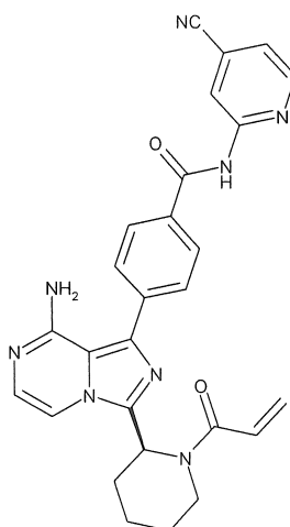
(S)-4-(3-(1-acryloylpiperidin-2-yl)-8-aminoimidazo[1,5-a]pyrazin-1-yl)-N-(4-cyanopyridin-2-yl)benzamidit
