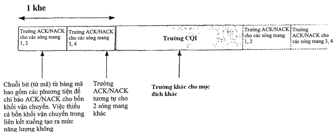
HARQ ACK cho 4 sóng mang + MIMO Rel-10
