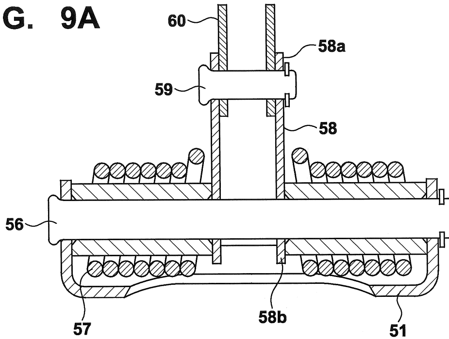
MẶT CẮT i-i
