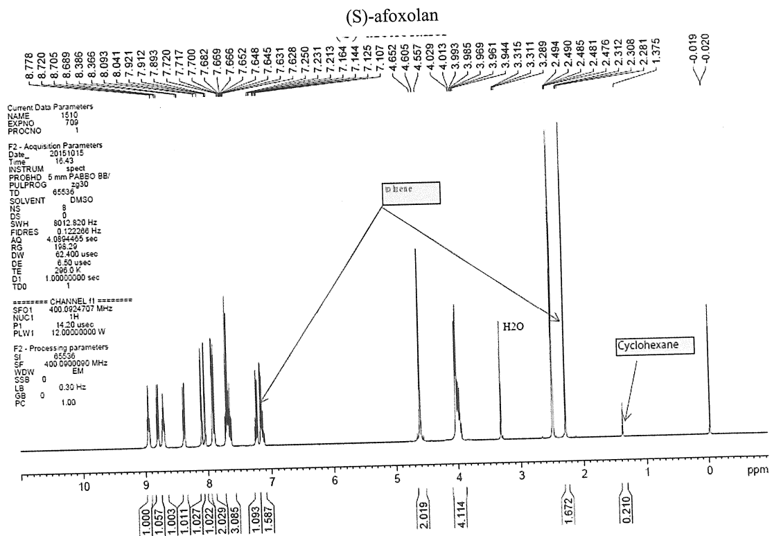
Fig. 3: ^1\text{H} NMR của (S)-afoxolan trong DMSO- \text{d}_6 được điều chế trong Ví dụ 7
