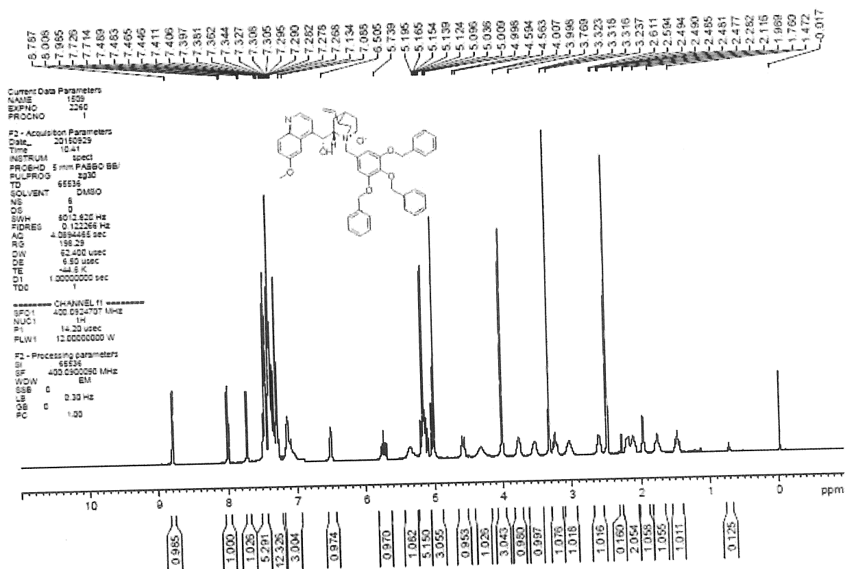
Fig. 1: Phổ ^1\text{H} NMR của chất xúc tác chuyển pha bất đối (IIIa-13-1) được điều chế trong Ví dụ 1 trong \text{DMSO-d}_6
