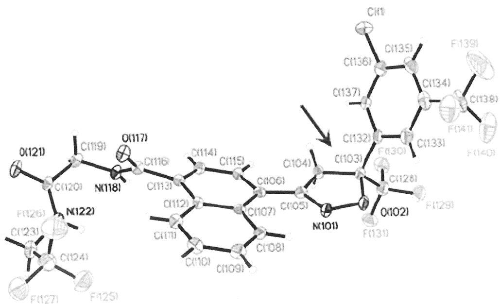
Fig. 10: Cấu trúc phân tử của ( S )-afloxolan từ phần mềm Cerius 2
