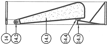
Mặt cắt F1-F1 Hình 54b
