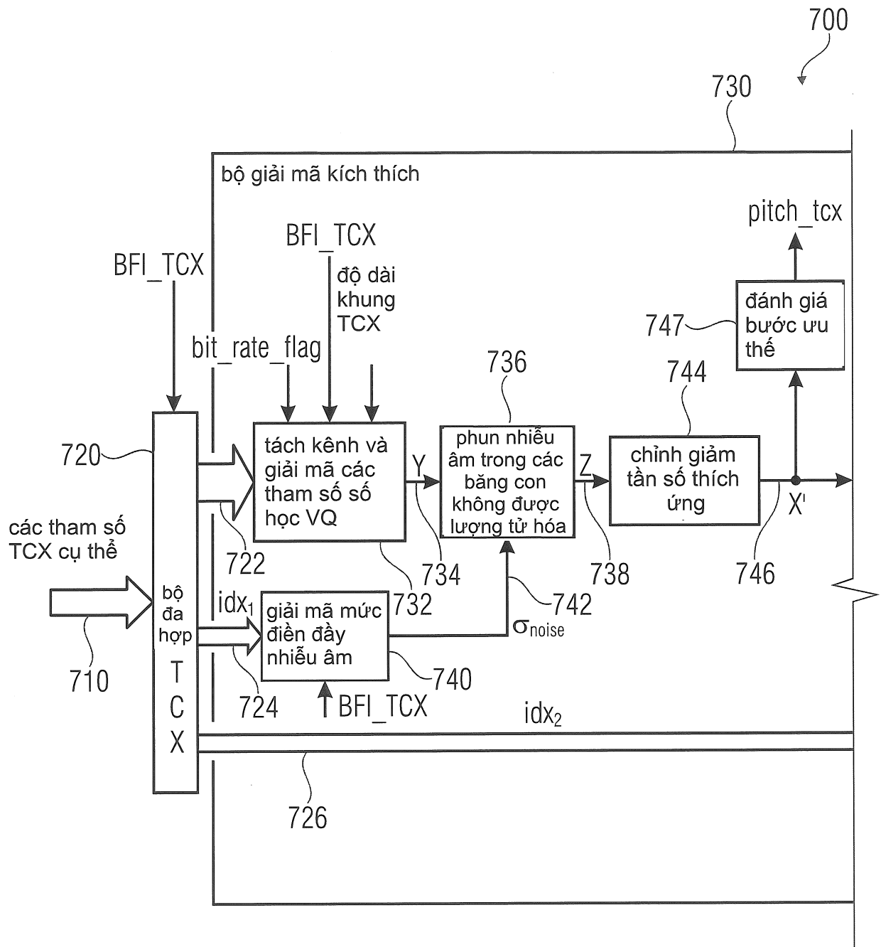
Sơ đồ khối của bộ giải mã TCX
