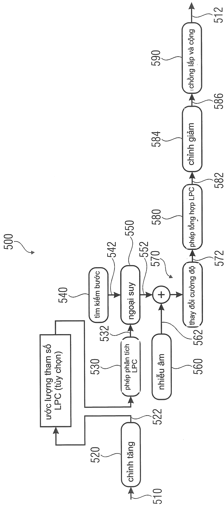
Tổng quan về sự che giấu miền thời gian cho bộ giải mã biến đổi
