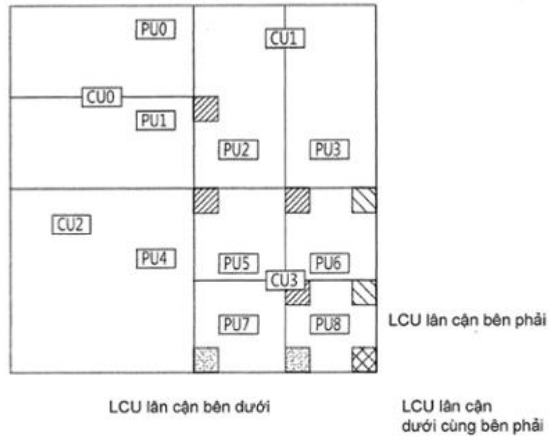
Phân chia CU/PU trong LCU hiện thời
